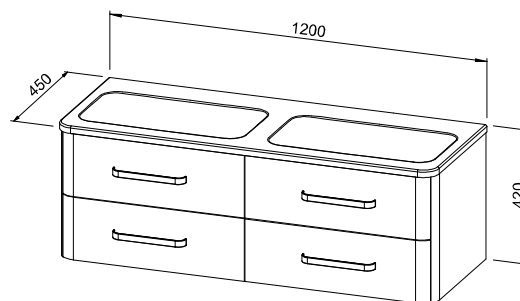
Baza s 4 ladice i umivaonikom Osnova z 4 predaloma in umivalnikom
