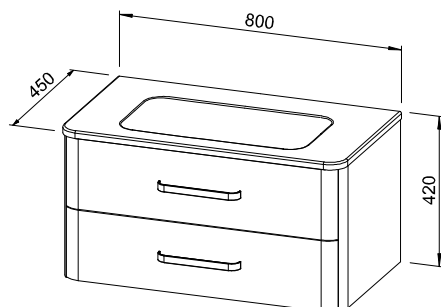
Baza s 2 ladice i umivaonikom Osnova z 2 predaloma in umivalnikom
