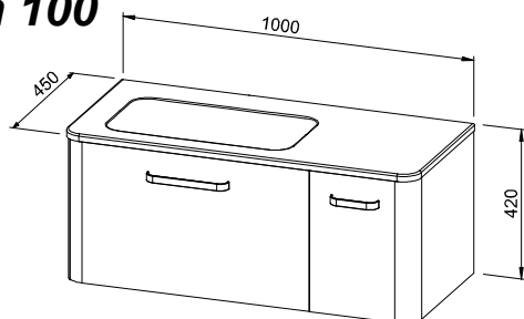
Baza s 2 ladice i umivaonikom Osnova z 2 predaloma in umivalnikom
