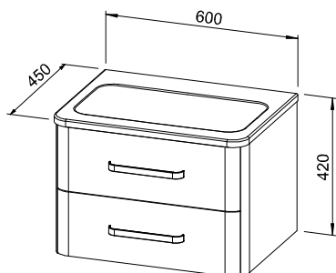
Baza s 2 ladice i umivaonikom Osnova z 2 predaloma in umivalnikom
