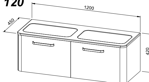
Baza s 2 ladice i umivaonikom Osnova z 2 predaloma in umivalnikom
