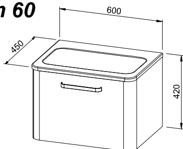
Baza s 1 ladicom i umivaonikom Osnova z 1 predalom in umivalnikom
