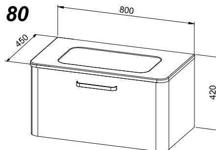
Baza s 1 ladicom i umivaonikom Osnova z 1 predalom in umivalnikom
