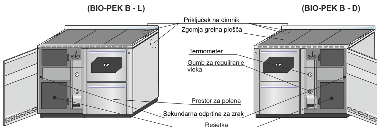
Slika 9. Osnovni deli
