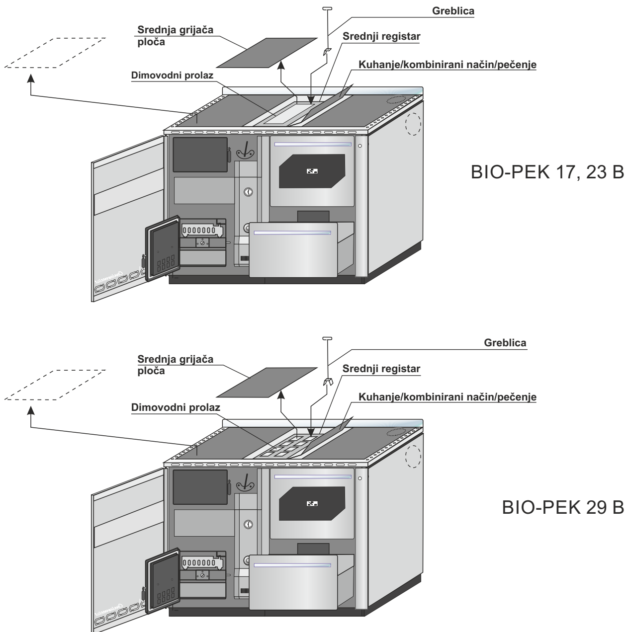
Slika 8. Čišćenje površina – kotao BIO-PEK B–D (vrijedi i za kotao BIO-PEK B–L)
