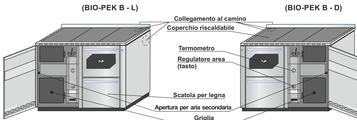
Foto 9. Componente generali
