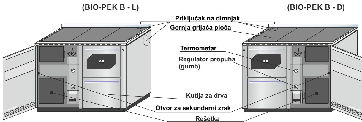
Slika 9. Osnovni dijelovi
