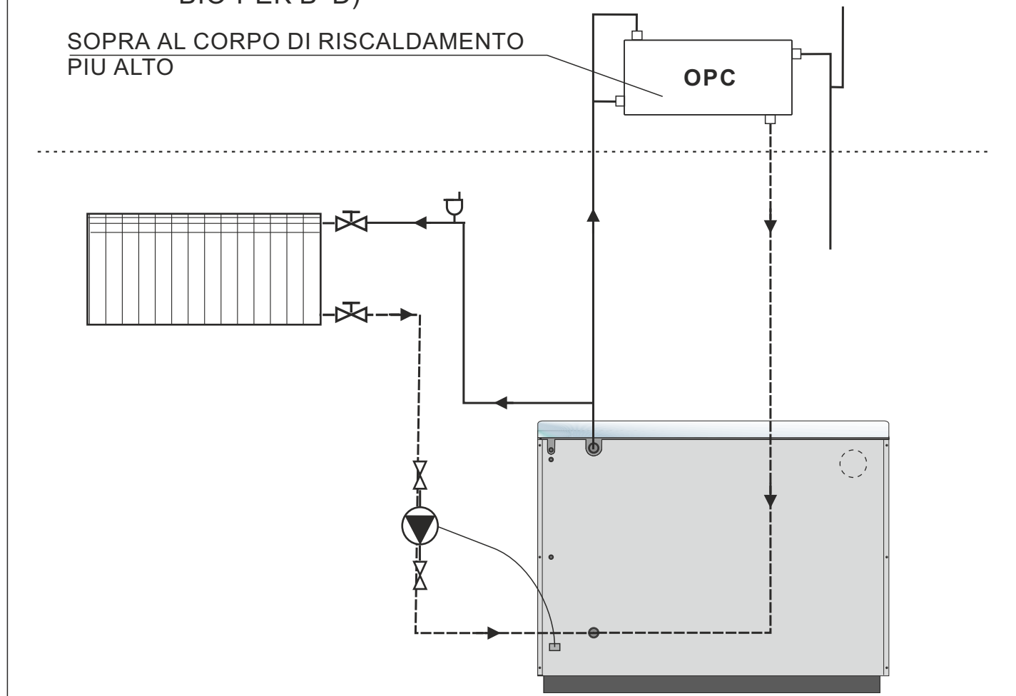
Schema 1: Collegamento della caldaia BIO-PEK B-L (vale anche per la caldaia BIO-PEK B-D)
